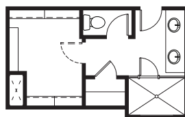
OPTIONAL GRAND MASTER SUITE 2
